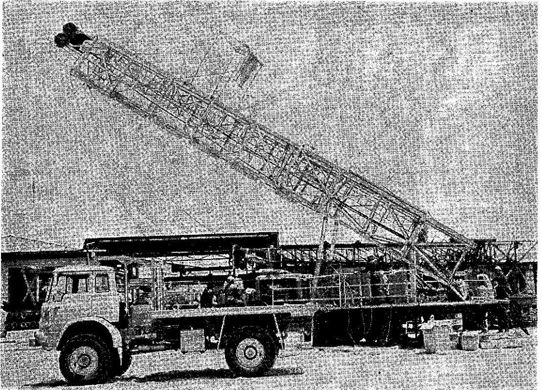
احدى آلات الشركة الحديثة ( ميهيو ٣٠٠٠ ) التي تستطيع ان تصل الى عمق ١٦٠٠ متر
